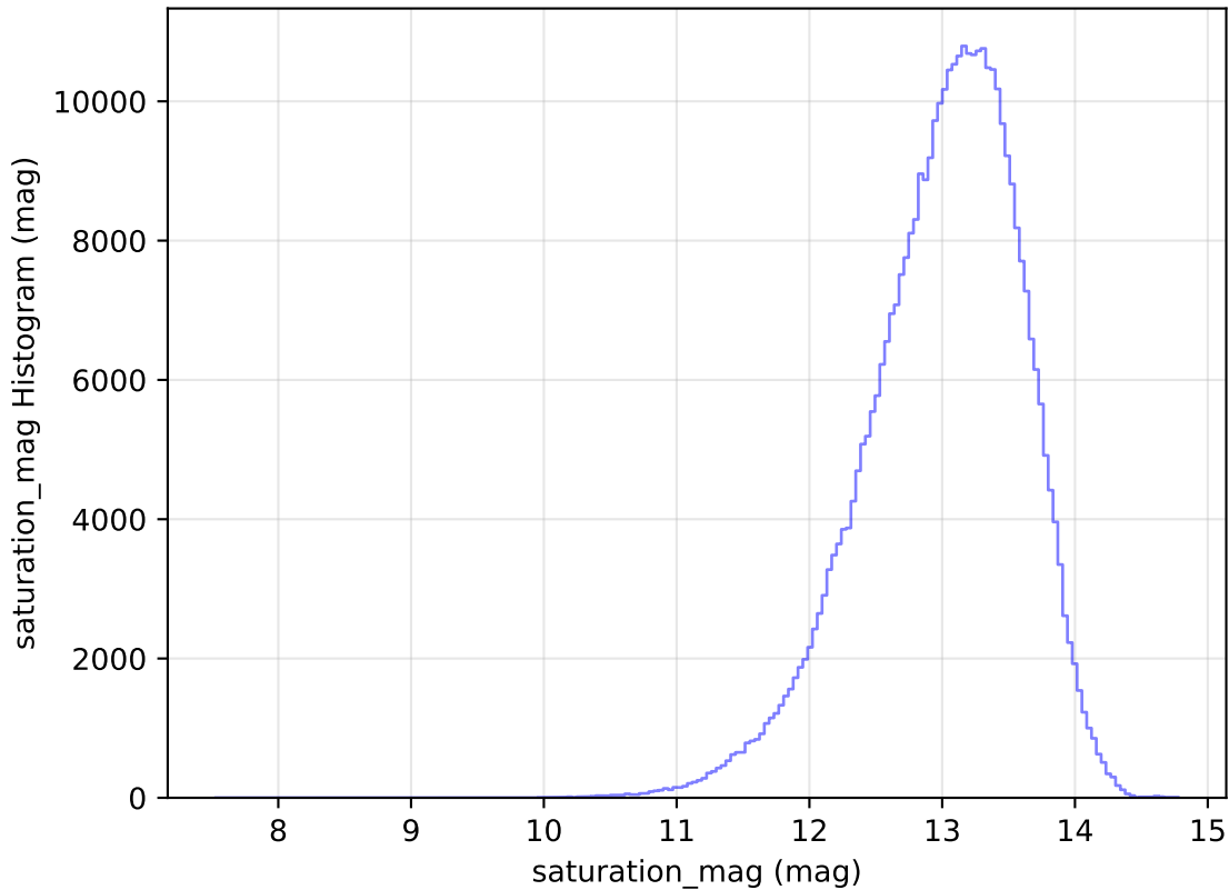
weather_cloudso20v3.4_10yrs All sky y band: saturation_mag Histogram
