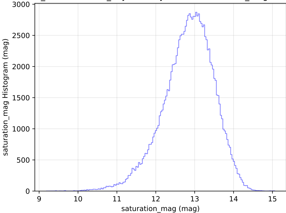
weather_cloudso20v3.4_10yrs All sky u band: saturation_mag Histogram
