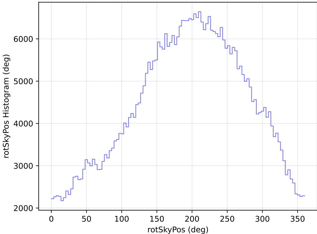
weather_cloudso20v3.4_10yrs WFD z band: rotSkyPos Histogram
