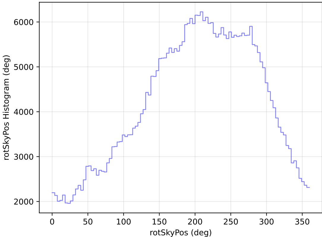
weather_cloudso20v3.4_10yrs WFD y band: rotSkyPos Histogram
