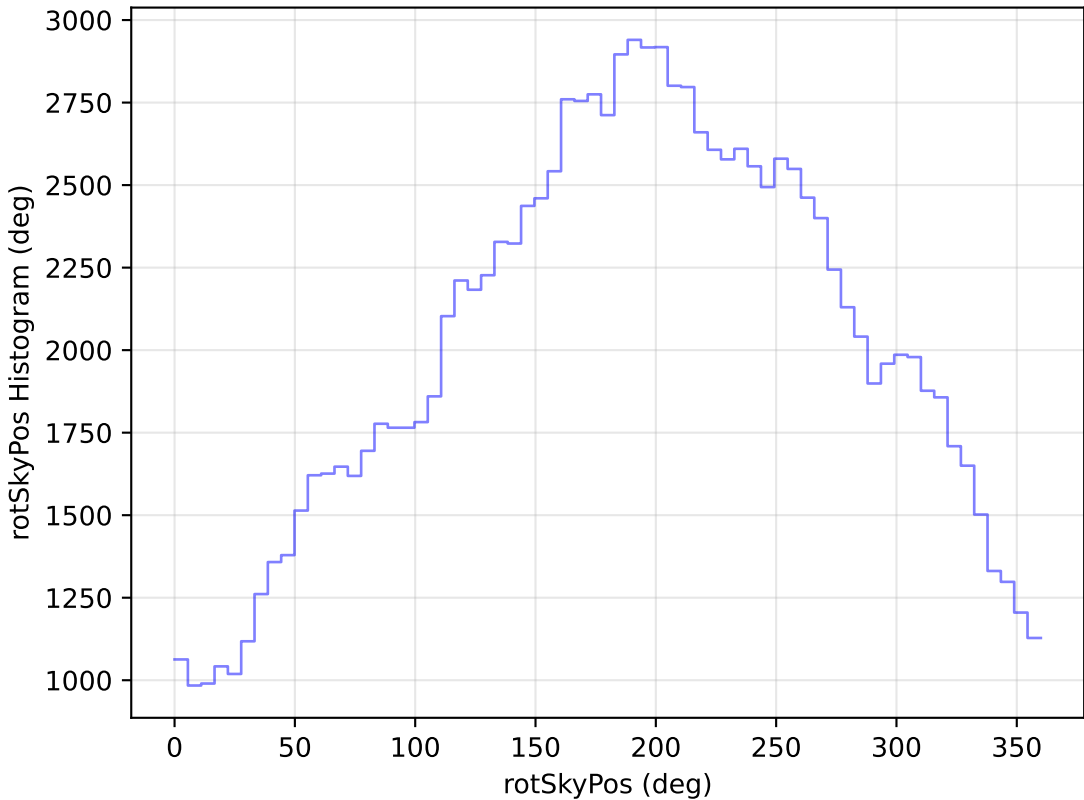
weather_cloudso20v3.4_10yrs WFD u band: rotSkyPos Histogram
