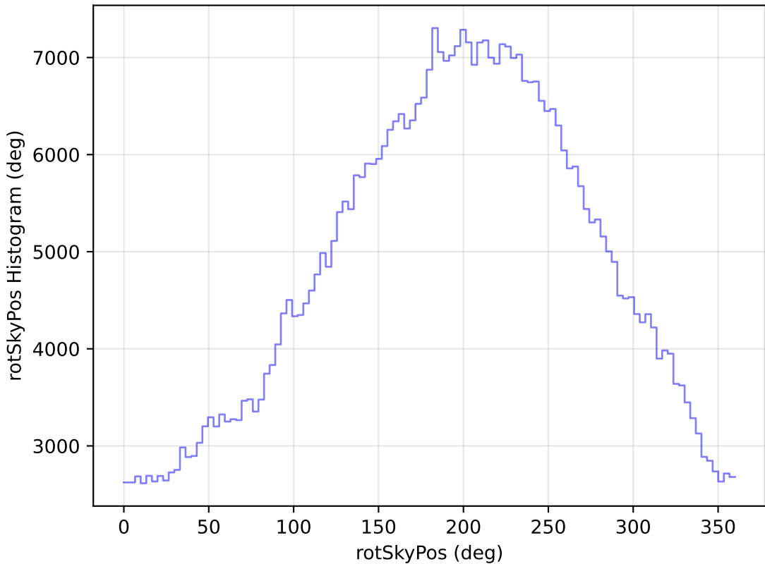
weather_cloudso20v3.4_10yrs WFD i band: rotSkyPos Histogram
