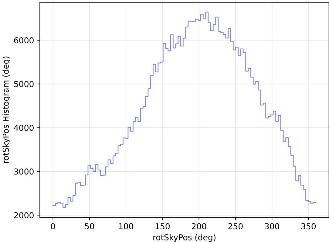
weather_cloudso20v3.4_10yrs All sky z band: rotSkyPos Histogram
