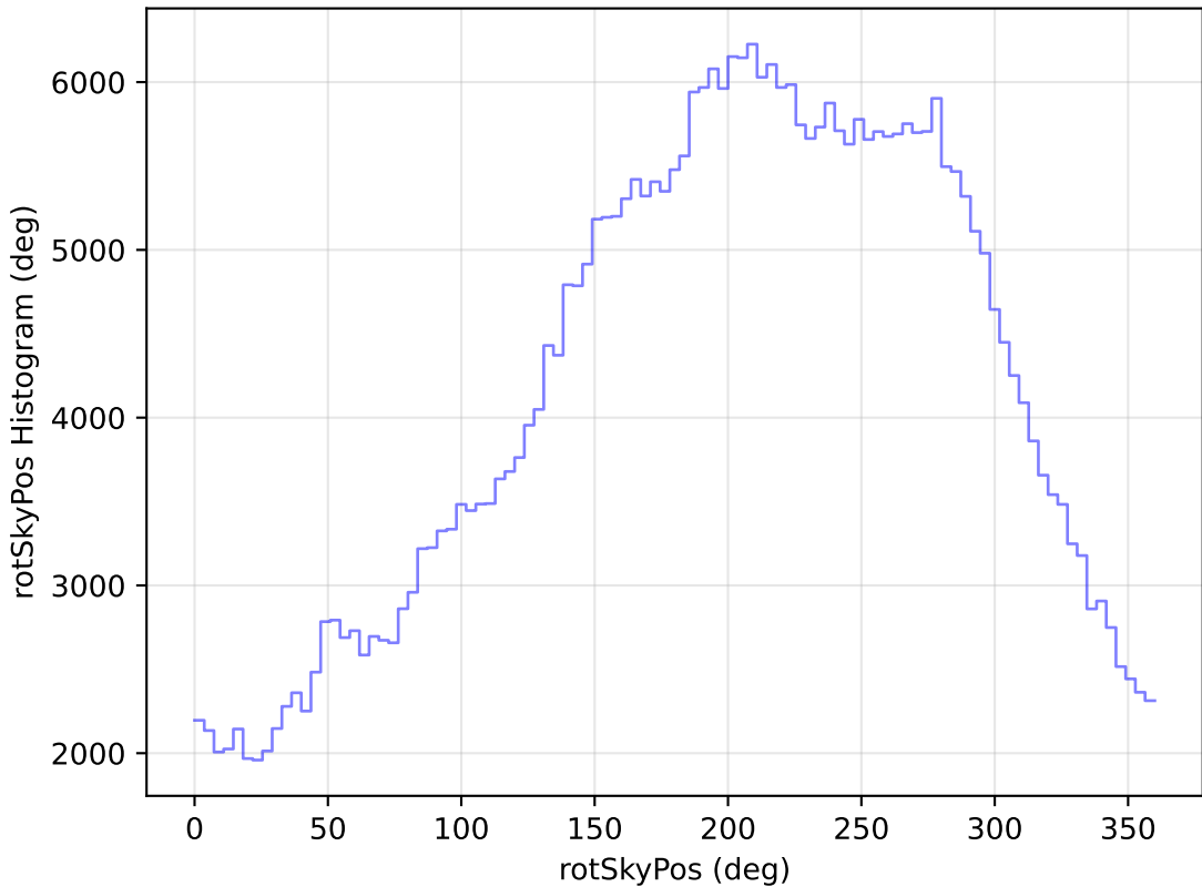
weather_cloudso20v3.4_10yrs All sky y band: rotSkyPos Histogram
