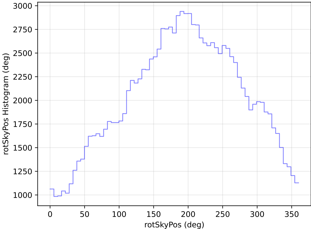
weather_cloudso20v3.4_10yrs All sky u band: rotSkyPos Histogram
