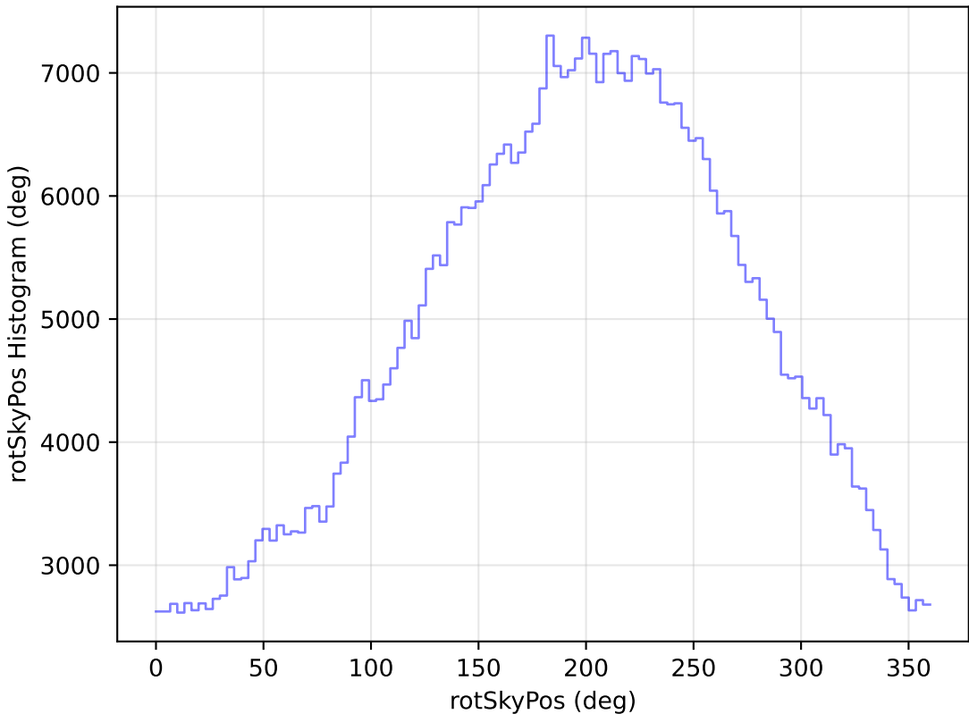
weather_cloudso20v3.4_10yrs All sky i band: rotSkyPos Histogram
