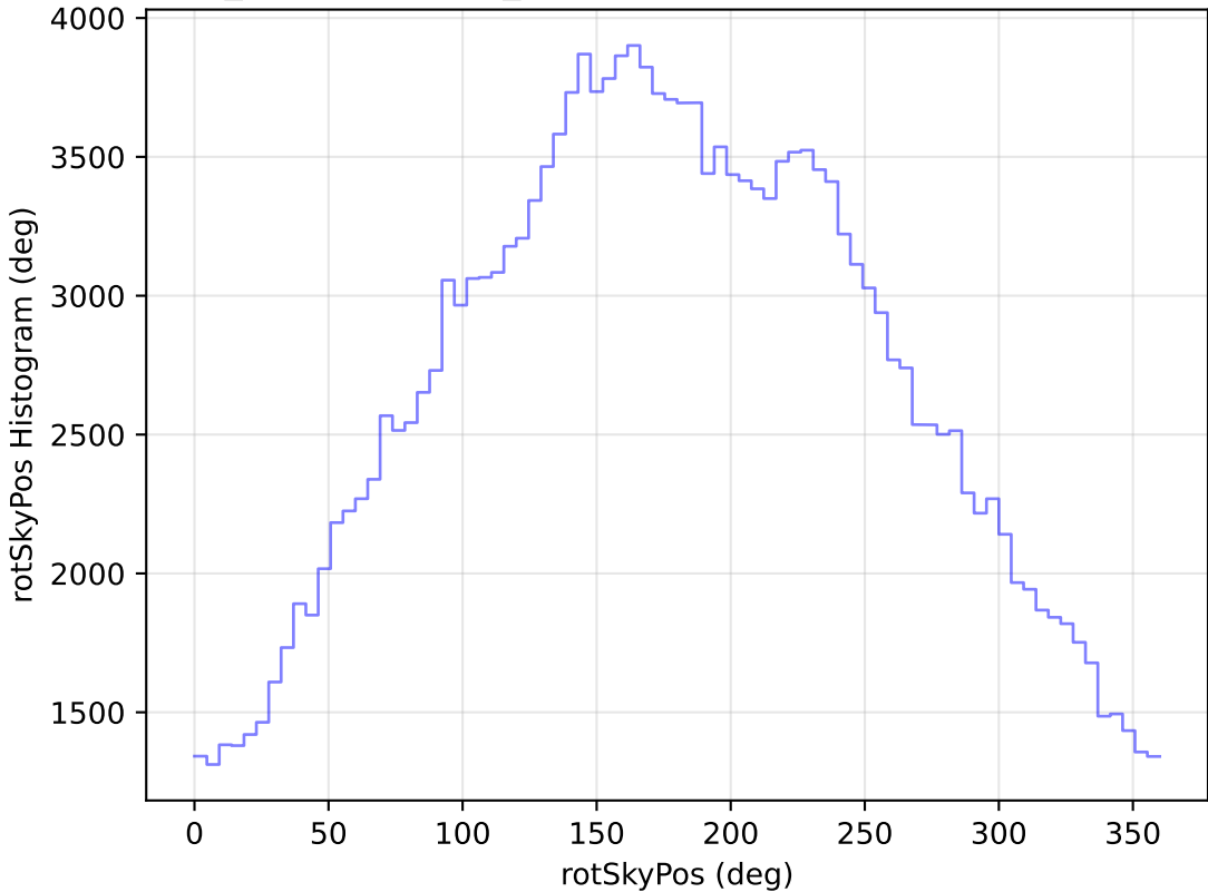
weather_cloudso20v3.4_10yrs All sky g band: rotSkyPos Histogram
