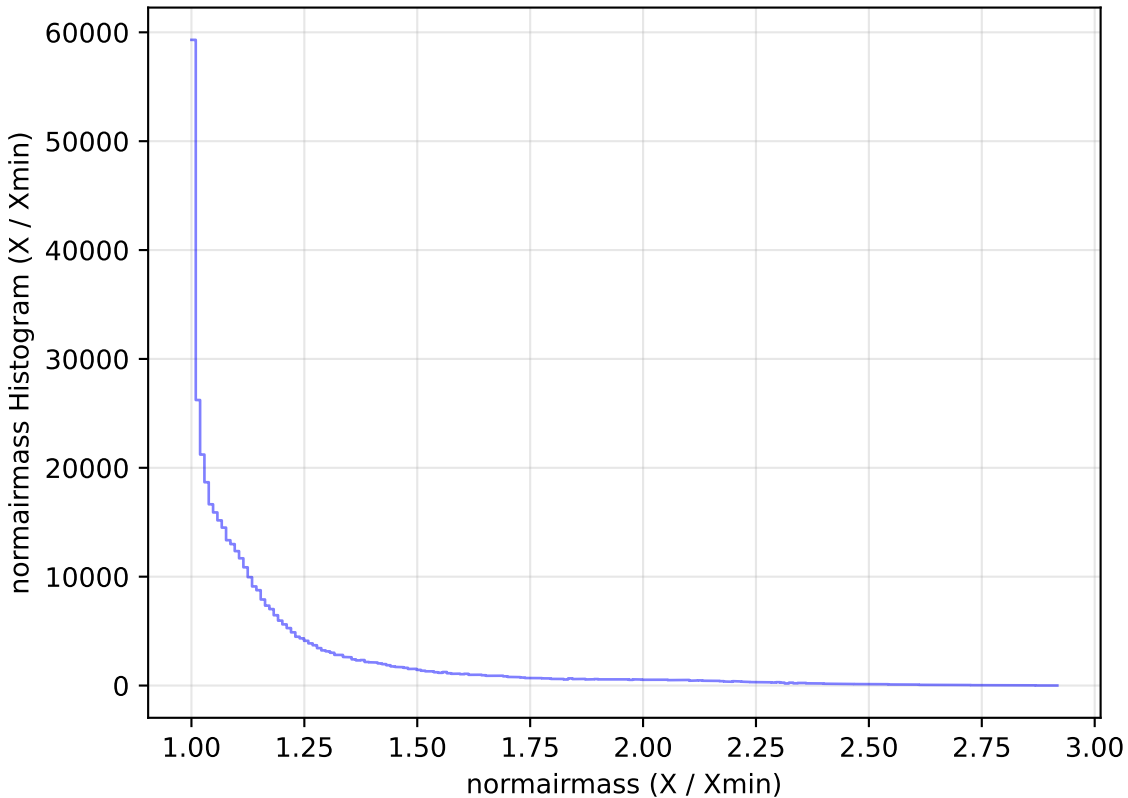
weather_cloudso20v3.4_10yrs WFD z band: normairmass Histogram
