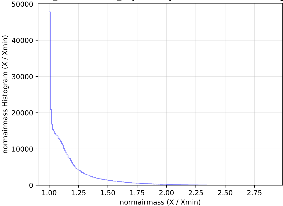
weather_cloudso20v3.4_10yrs WFD y band: normairmass Histogram
