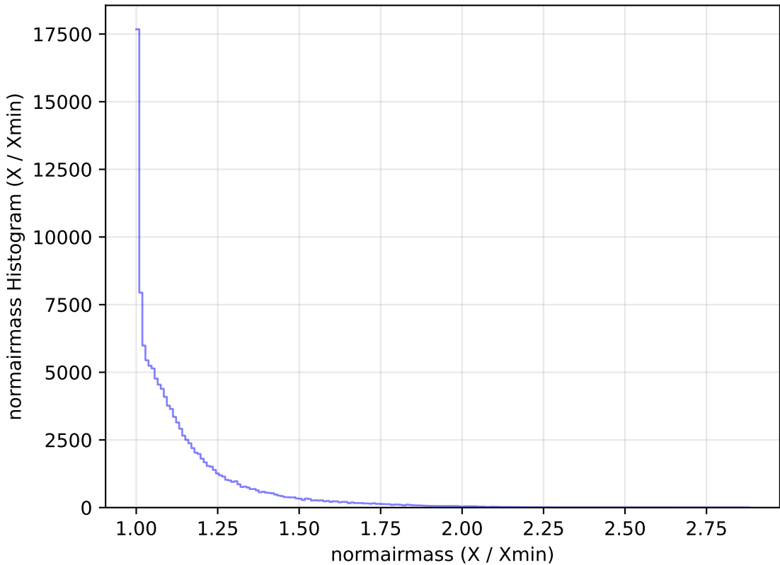
weather_cloudso20v3.4_10yrs WFD u band: normairmass Histogram
