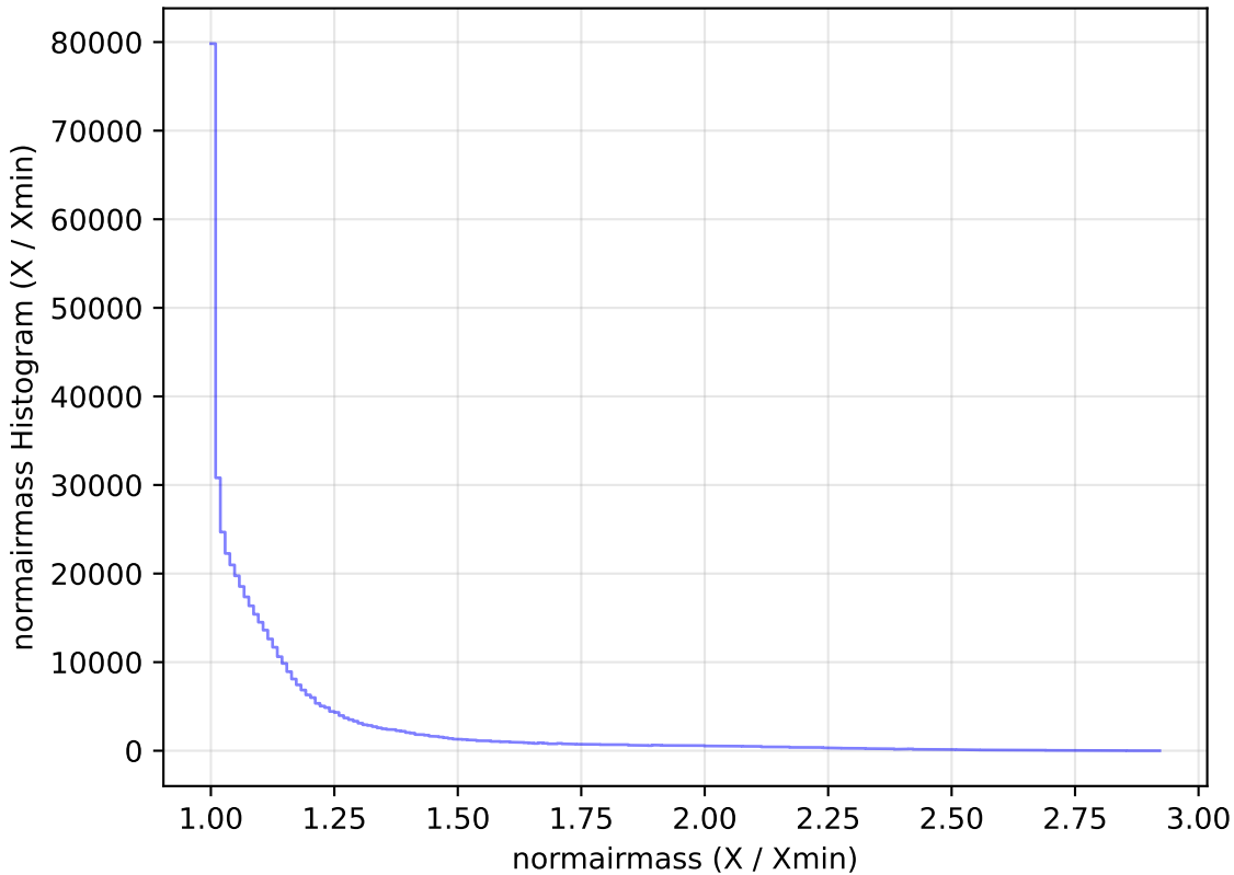
weather_cloudso20v3.4_10yrs WFD i band: normairmass Histogram
