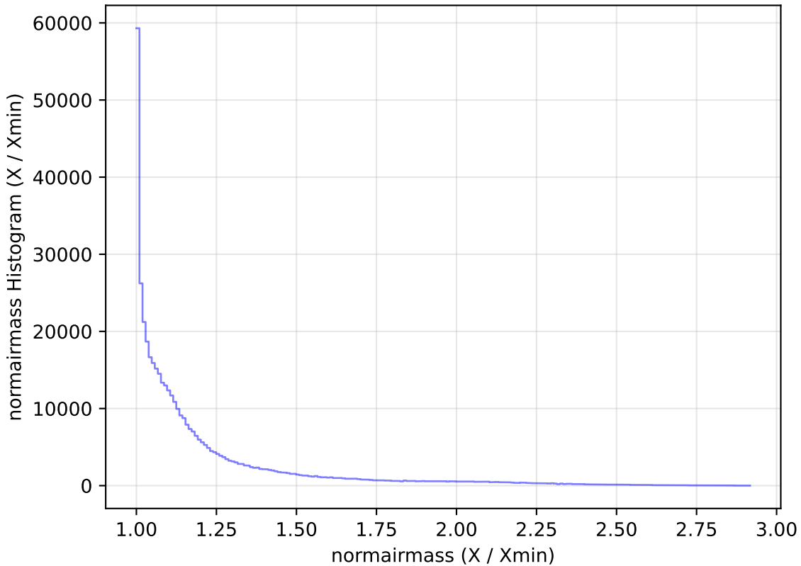
weather_cloudso20v3.4_10yrs All sky z band: normairmass Histogram
