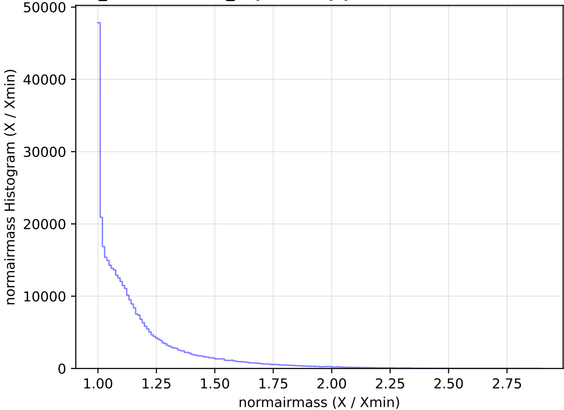
weather_cloudso20v3.4_10yrs All sky y band: normairmass Histogram
