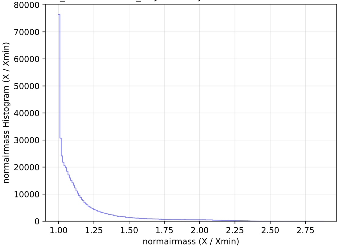
weather_cloudso20v3.4_10yrs All sky r band: normairmass Histogram
