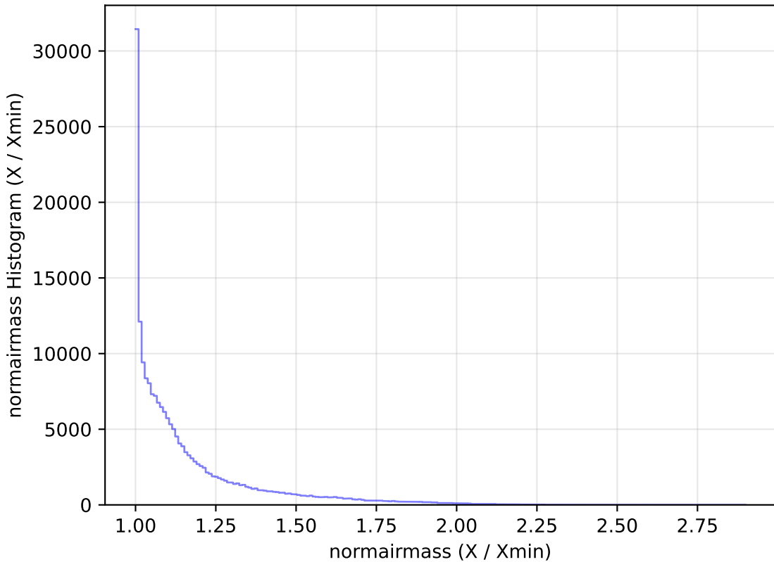
weather_cloudso20v3.4_10yrs All sky g band: normairmass Histogram
