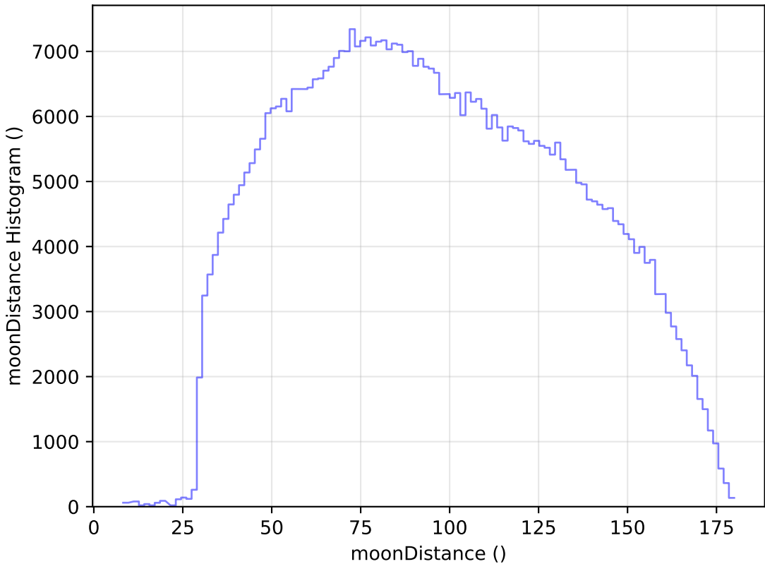
weather_cloudso20v3.4_10yrs WFD i band: moonDistance Histogram
