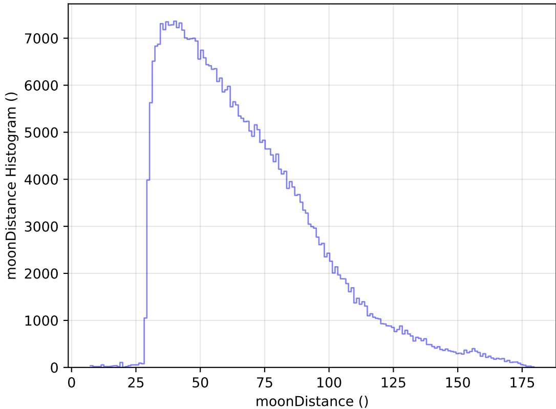
weather_cloudso20v3.4_10yrs All sky y band: moonDistance Histogram
