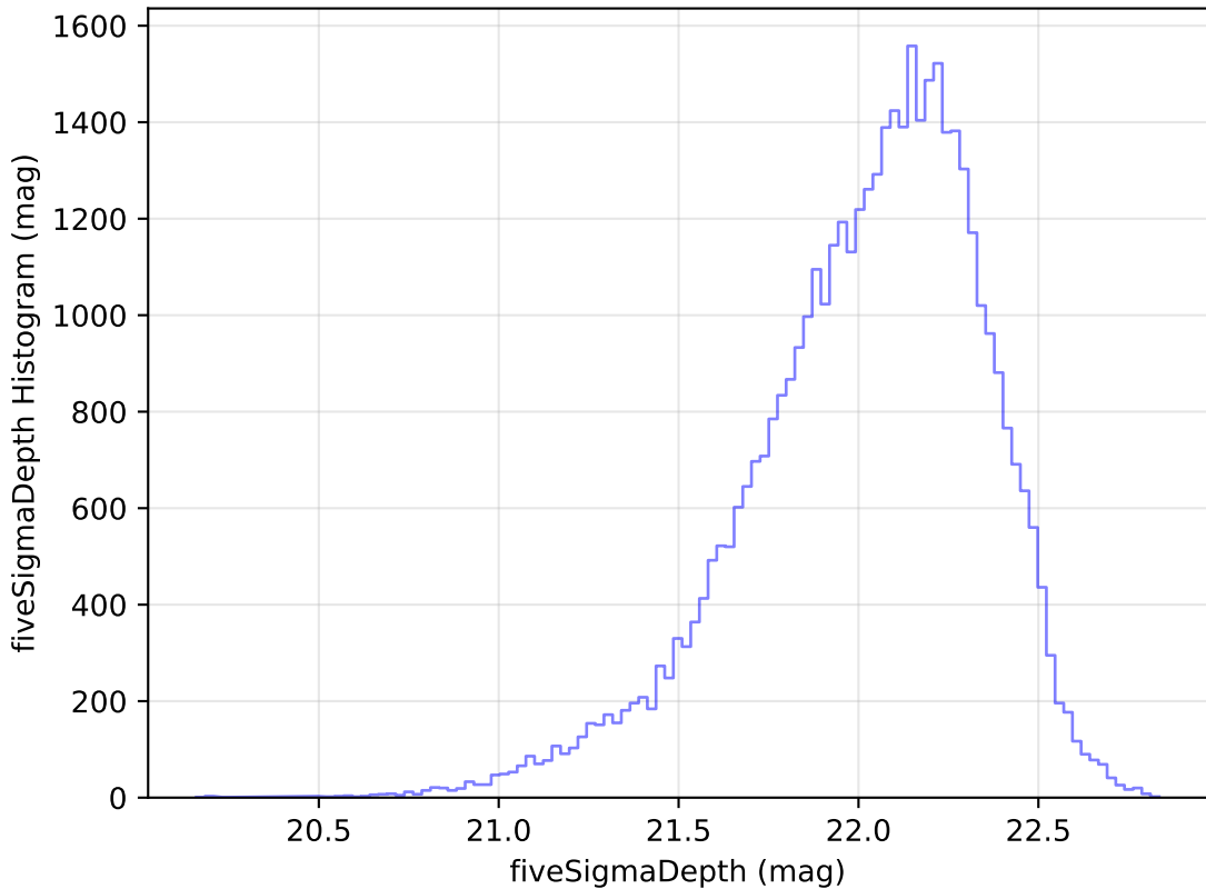
weather_cloudso20v3.4_10yrs Yr 1 y band: fiveSigmaDepth Histogram
