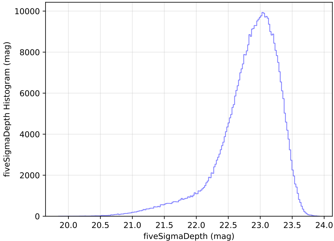
weather_cloudso20v3.4_10yrs WFD z band: fiveSigmaDepth Histogram
