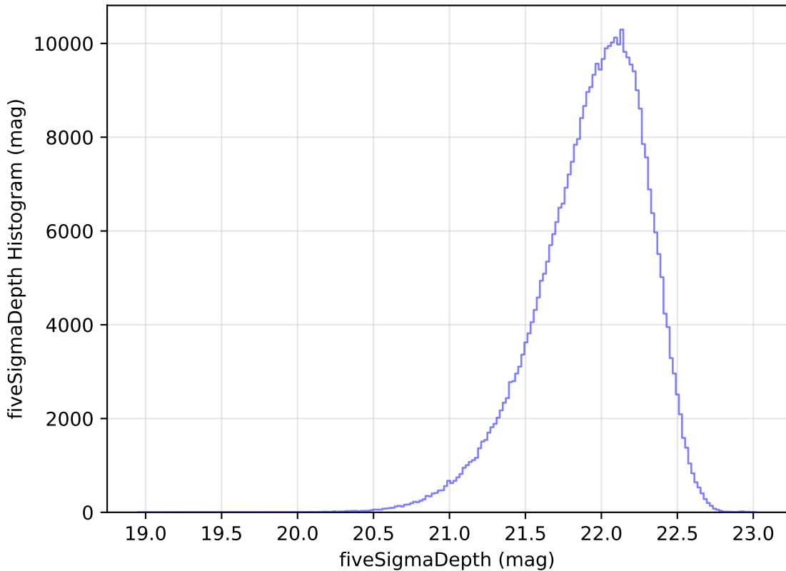
weather_cloudso20v3.4_10yrs WFD y band: fiveSigmaDepth Histogram
