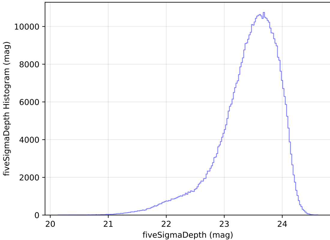
weather_cloudso20v3.4_10yrs All sky i band: fiveSigmaDepth Histogram
