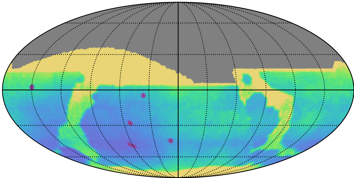
weather_cloudso20v3.4_10yrs All sky: Parallax Uncert @ 24.0
