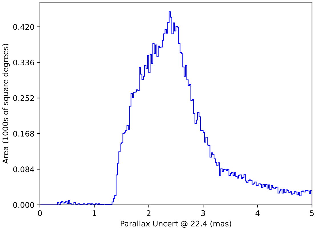
weather_cloudso20v3.4_10yrs All sky: Parallax Uncert @ 22.4
