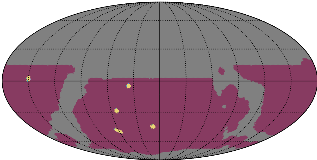
weather_cloudso20v3.4_10yrs WFD: NumberOfQuickRevisits
