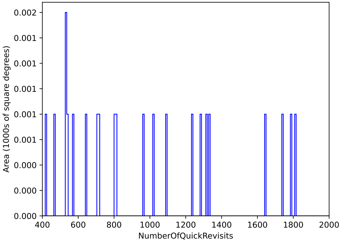
weather_cloudso20v3.4_10yrs WFD: NumberOfQuickRevisits
