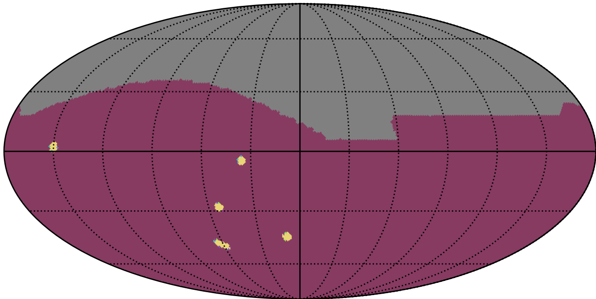
weather_cloudso20v3.4_10yrs All sky: NumberOfQuickRevisits
