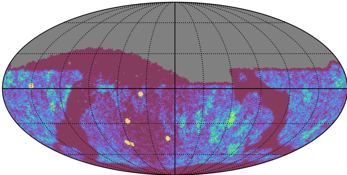
weather_cloudso20v3.4_10yrs Yr 1 z band: NVisits
