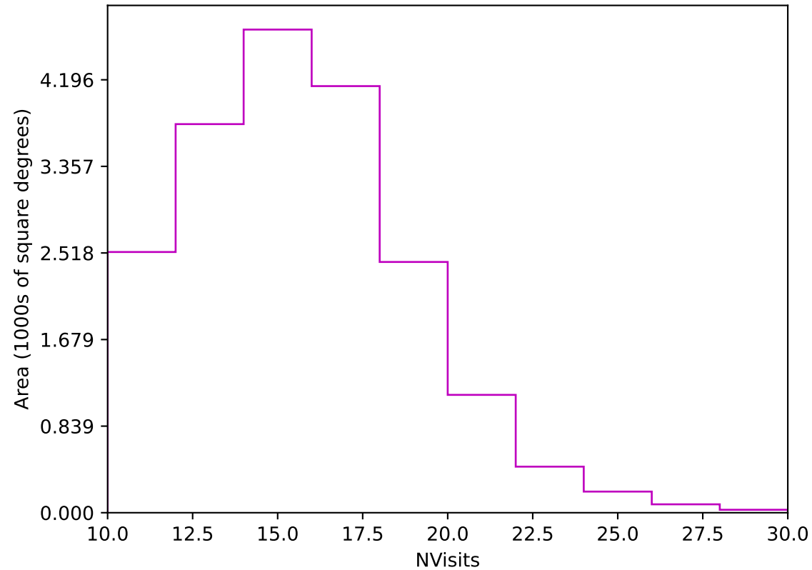
weather_cloudso20v3.4_10yrs Yr 1 z band: NVisits
