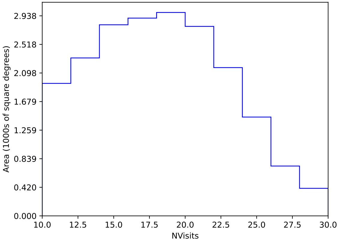
weather_cloudso20v3.4_10yrs Yr 1 y band: NVisits
