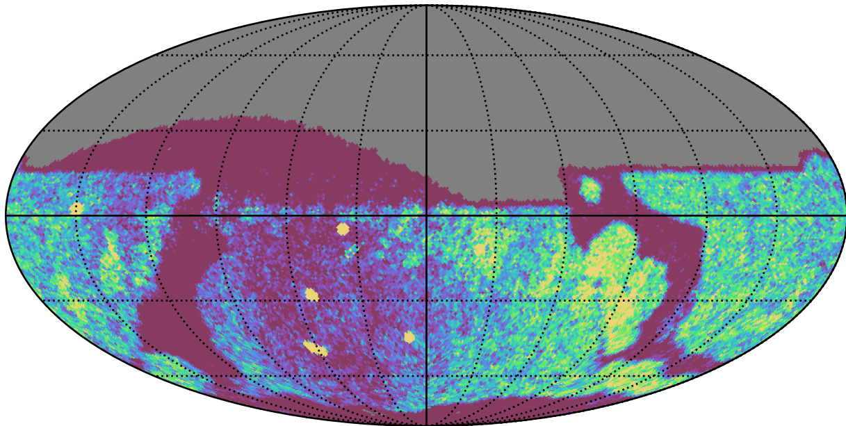
weather_cloudso20v3.4_10yrs Yr 1 r band: NVisits
