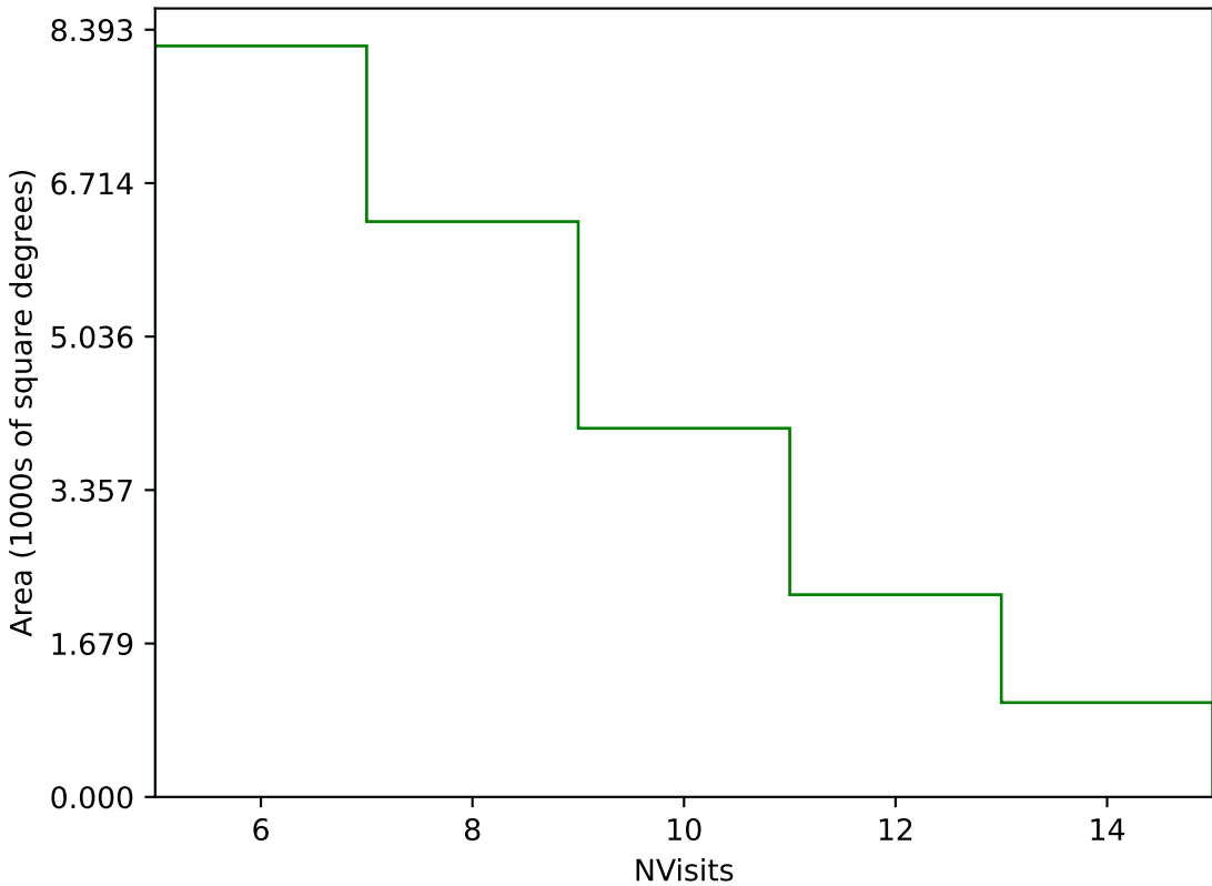
weather_cloudso20v3.4_10yrs Yr 1 g band: NVisits
