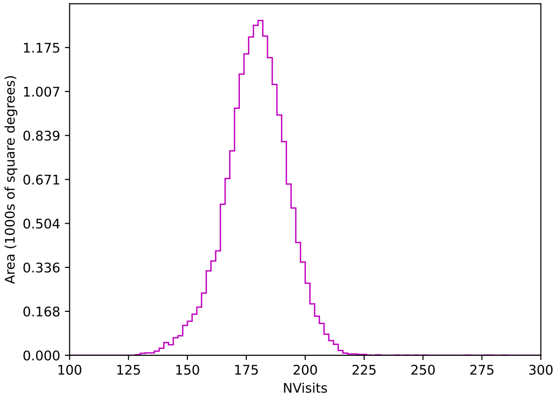
weather_cloudso20v3.4_10yrs WFD z band: NVisits
