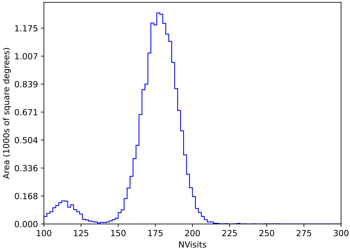
weather_cloudso20v3.4_10yrs WFD y band: NVisits
