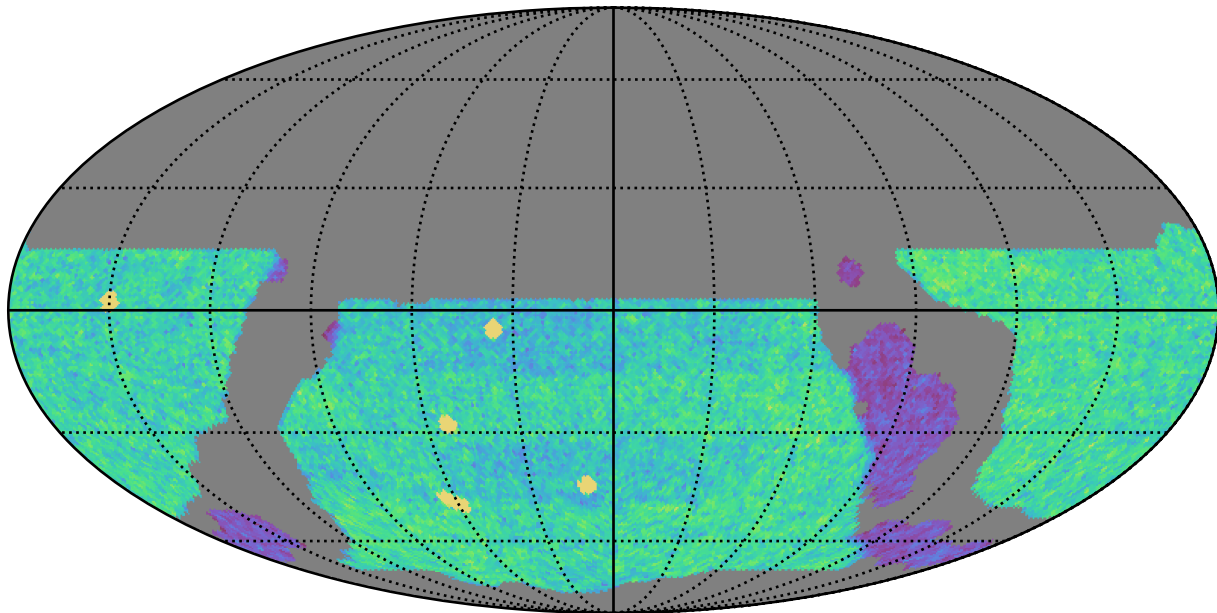
weather_cloudso20v3.4_10yrs WFD u band: NVisits
