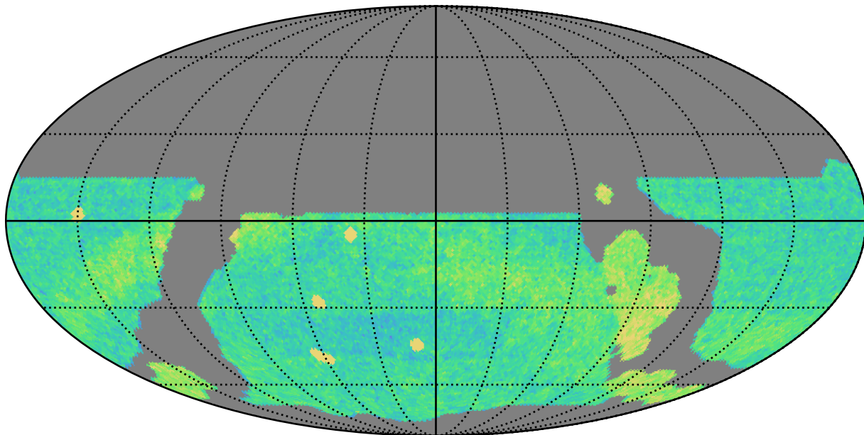
weather_cloudso20v3.4_10yrs WFD r band: NVisits
