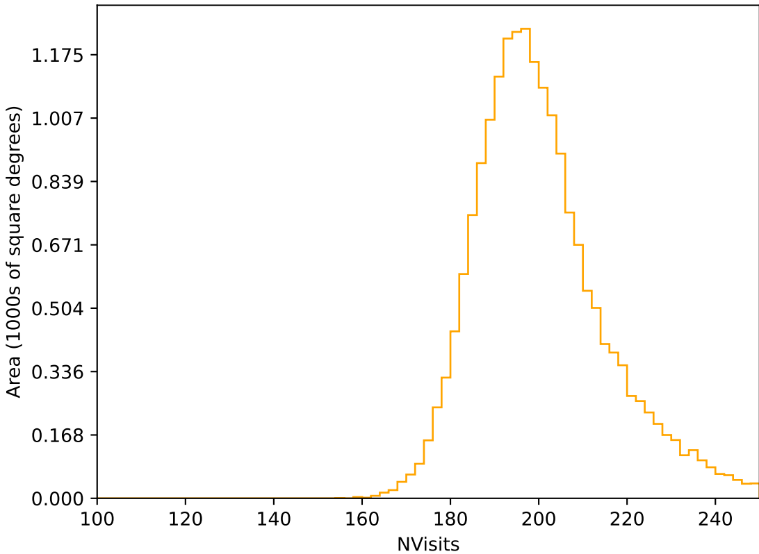
weather_cloudso20v3.4_10yrs WFD r band: NVisits
