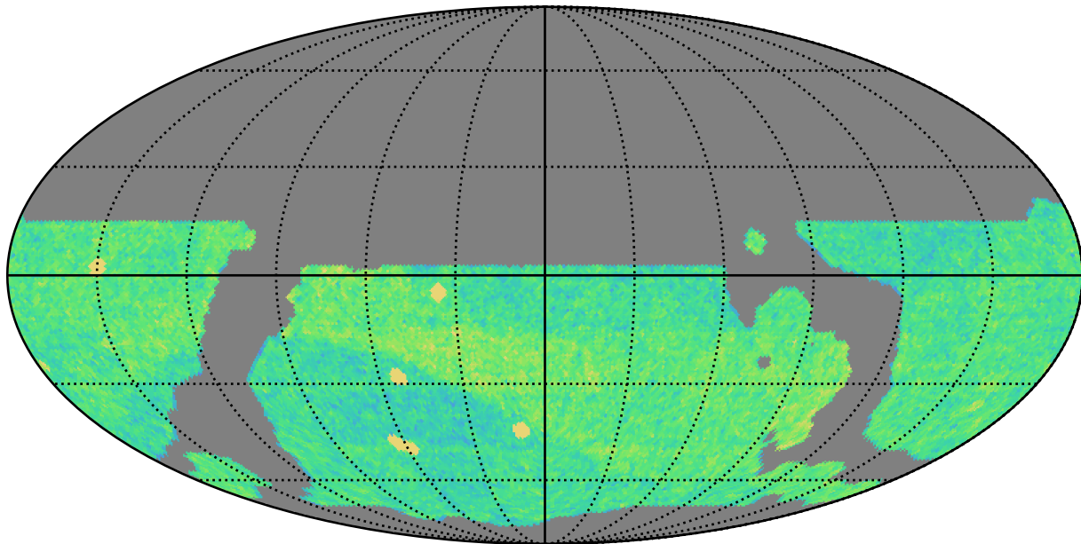
weather_cloudso20v3.4_10yrs WFD i band: NVisits
