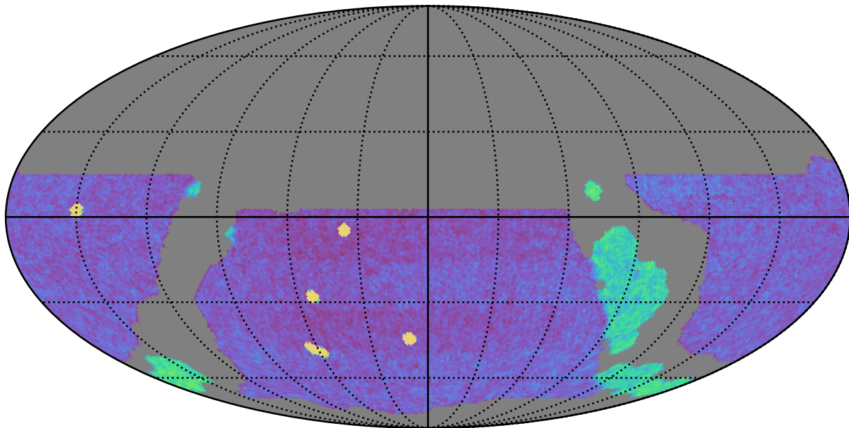
weather_cloudso20v3.4_10yrs WFD g band: NVisits
