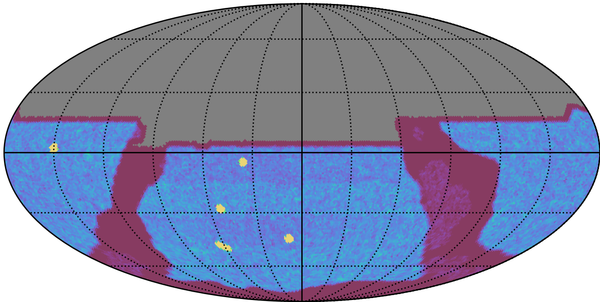
weather_cloudso20v3.4_10yrs All sky y band: NVisits
