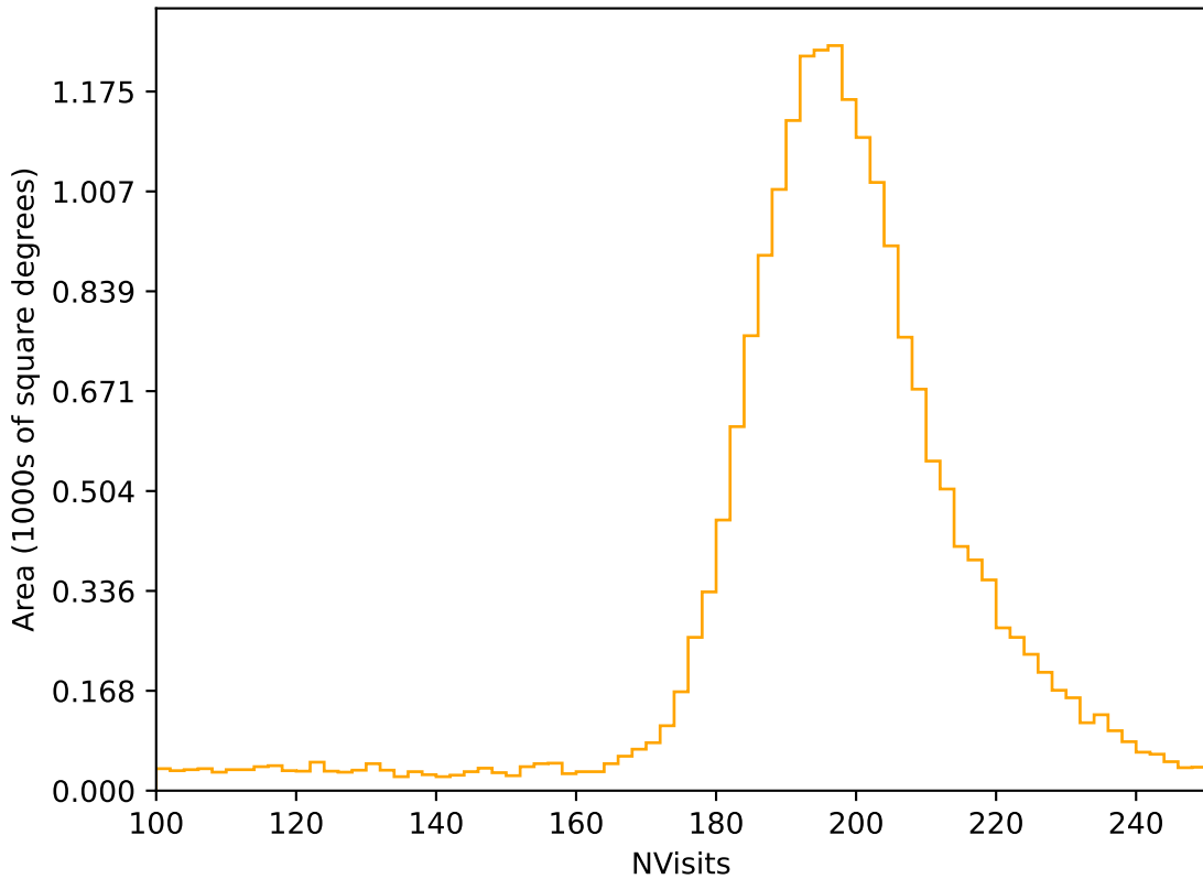
weather_cloudso20v3.4_10yrs All sky r band: NVisits
