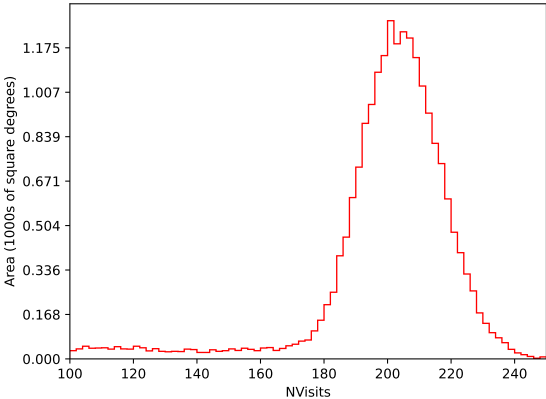
weather_cloudso20v3.4_10yrs All sky i band: NVisits
