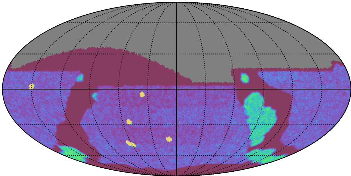
weather_cloudso20v3.4_10yrs All sky g band: NVisits
