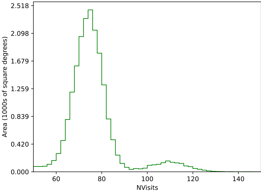
weather_cloudso20v3.4_10yrs All sky g band: NVisits
