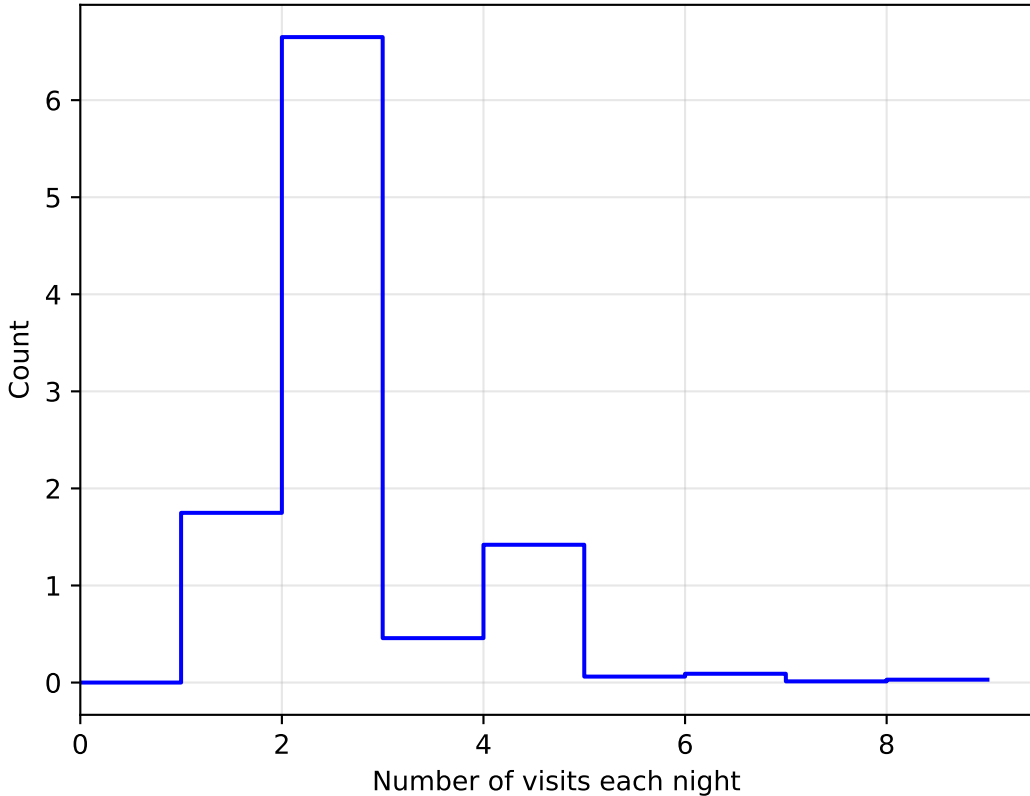
weather_cloudso20v3.4_10yrs All sky: NVisitsPerNight
