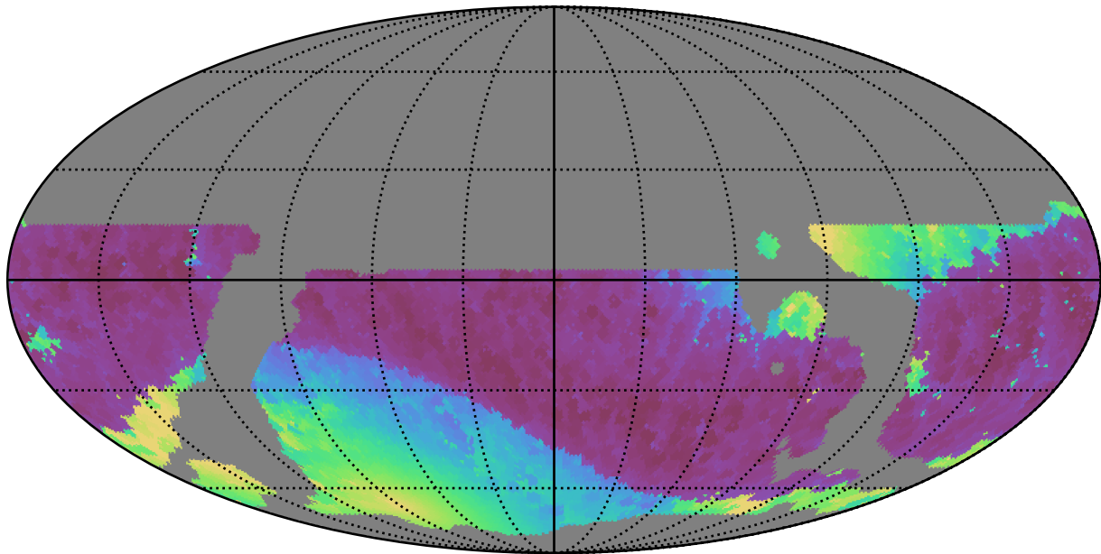
weather_cloudso20v3.4_10yrs WFD z band: Min solarElong
