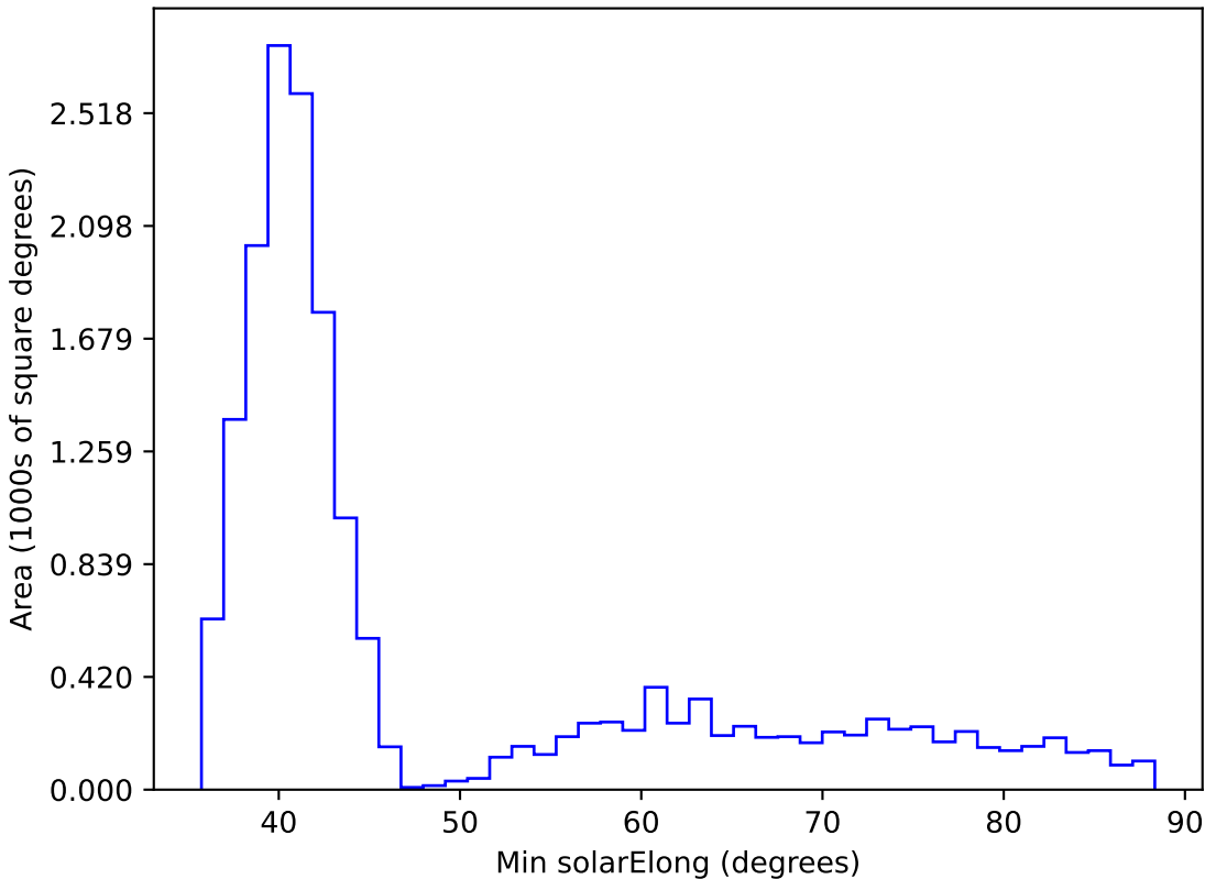
weather_cloudso20v3.4_10yrs WFD z band: Min solarElong
